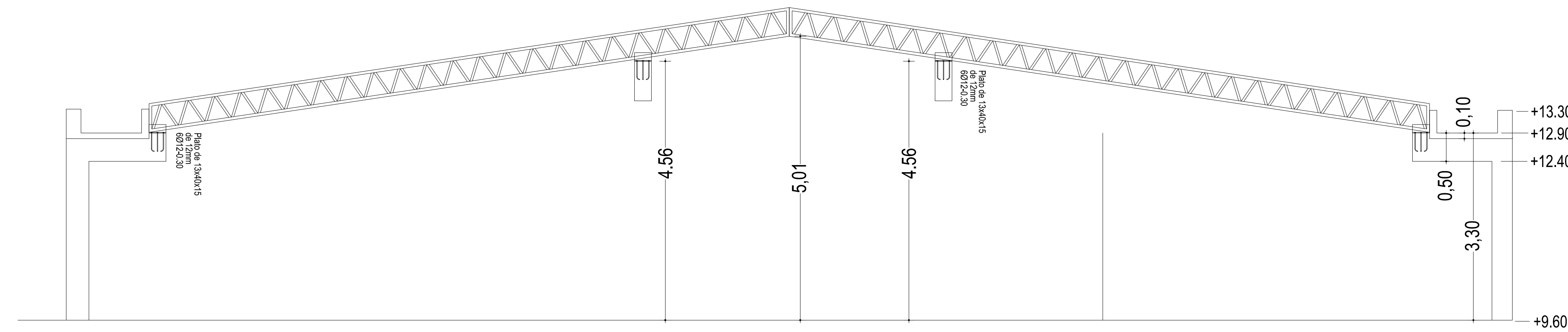
CORTE B-B
